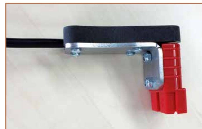
Ladestecker mit Zugentlastung und Griff
