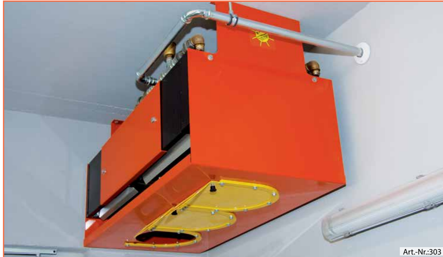
Kompakter Wärmetauscher zur Anwärmung der Ansaugluft
